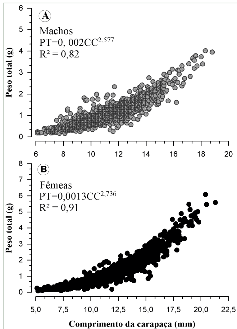
Figura 3. Relação biométrica de peso-comprimento para machos (A) e fêmeas (B) de M. amazonicum , coletados na ilha Tabatinga, Abaetetuba (PA).
